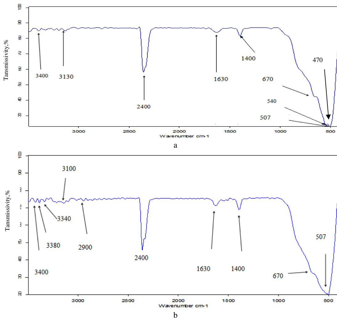
Fig. 3. TiO 2 transmission spectra: a – TiO 2 ; b – Ni-N-TiO 2
