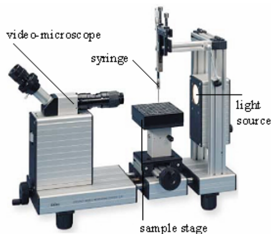
Fig. 2. Contact Angle Meter G10
